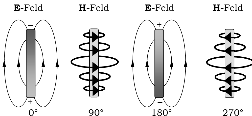
Bild 8: Die Felder der schwingende Dipolantenne
