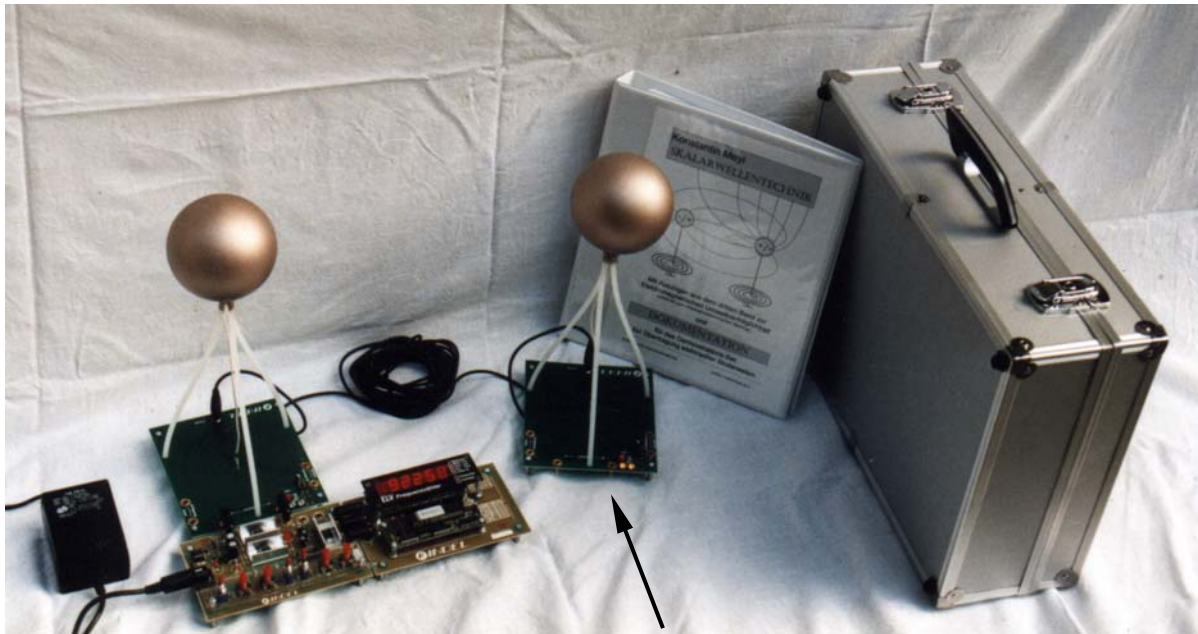
Netzgerät Sender (LED aus) Empfänger (2 LED leuchten!) Sinusgenerator + Frequenzzähler Dokumentation + Alukoffer
